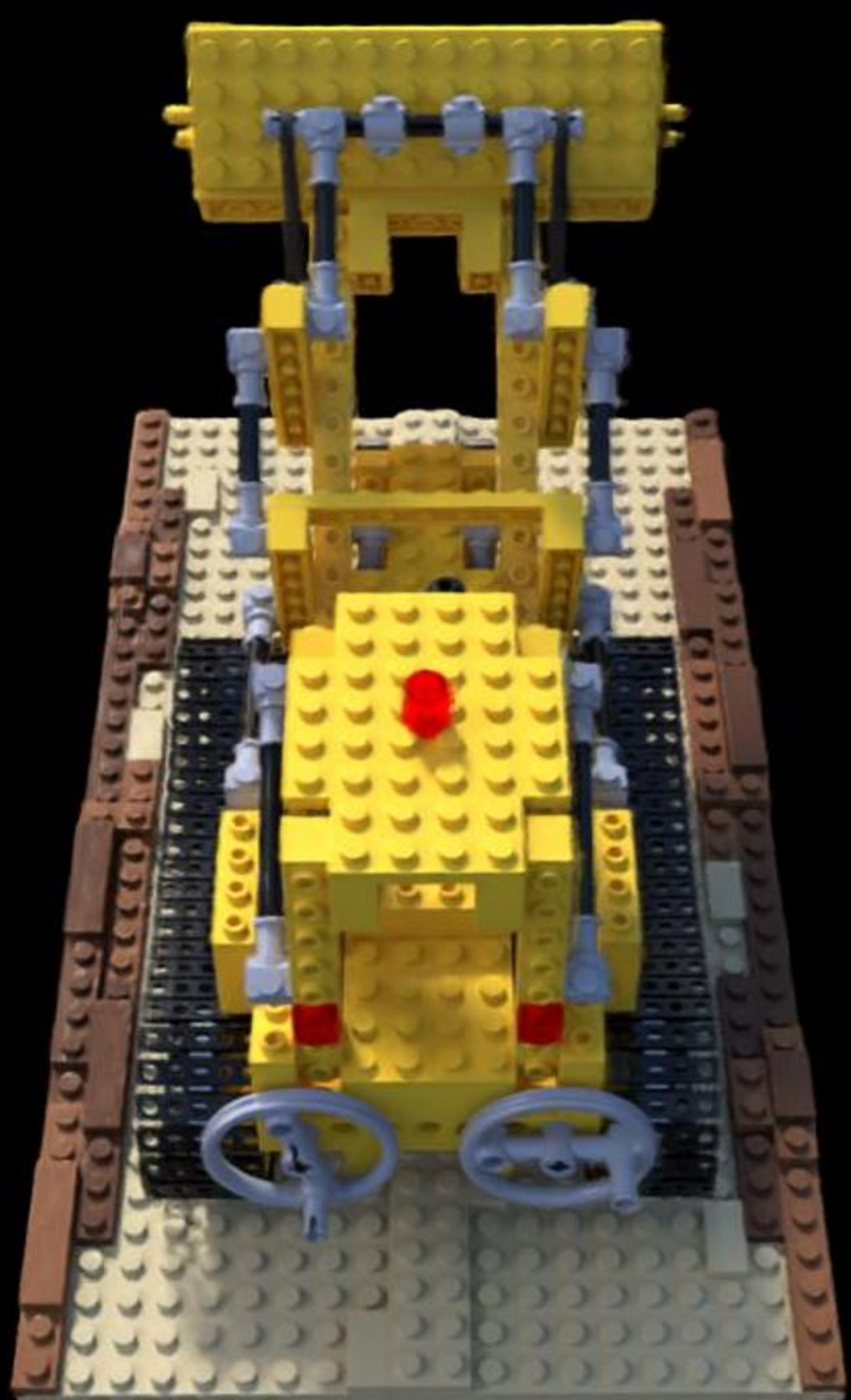
Config: VGGT | random | num_points=87000 PSNR: 19.91 | LPIPS: 0.1066 | SSIM: 0.7478
