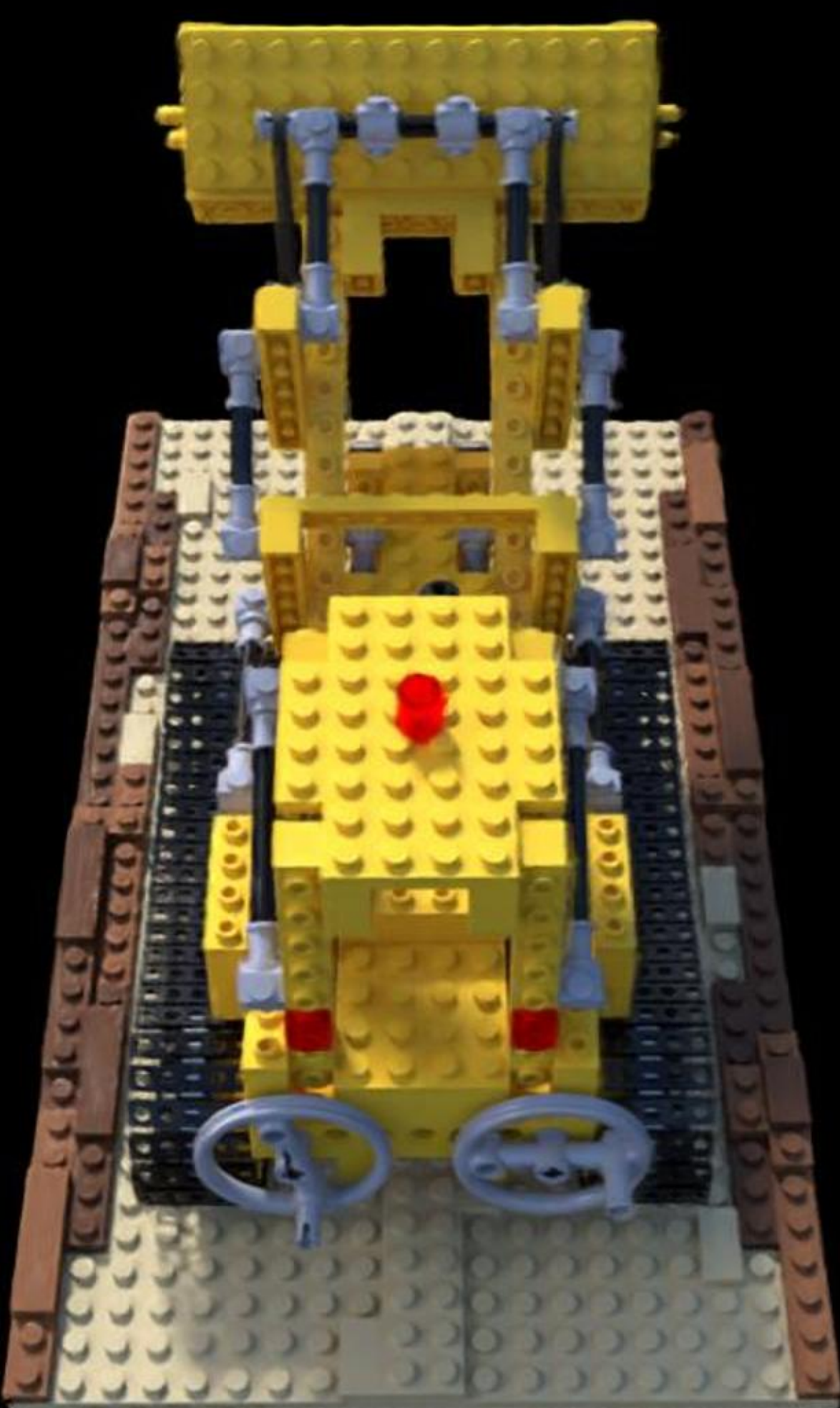
Config: VGGT | voxels | num_points=87000 PSNR: 19.85 | LPIPS: 0.1075 | SSIM: 0.7468
