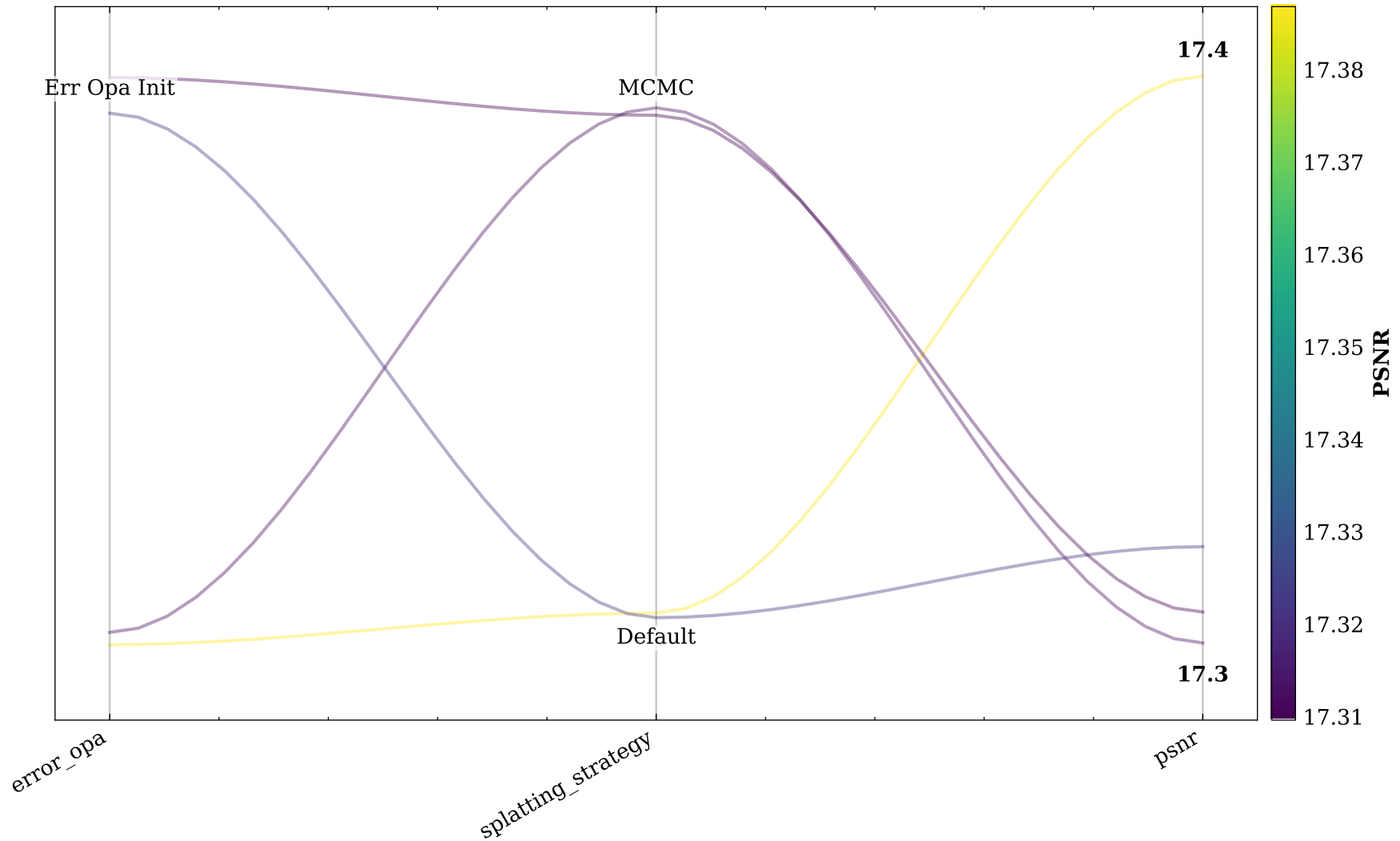
Parallel Coordinate Plot: Parameters vs PSNR
