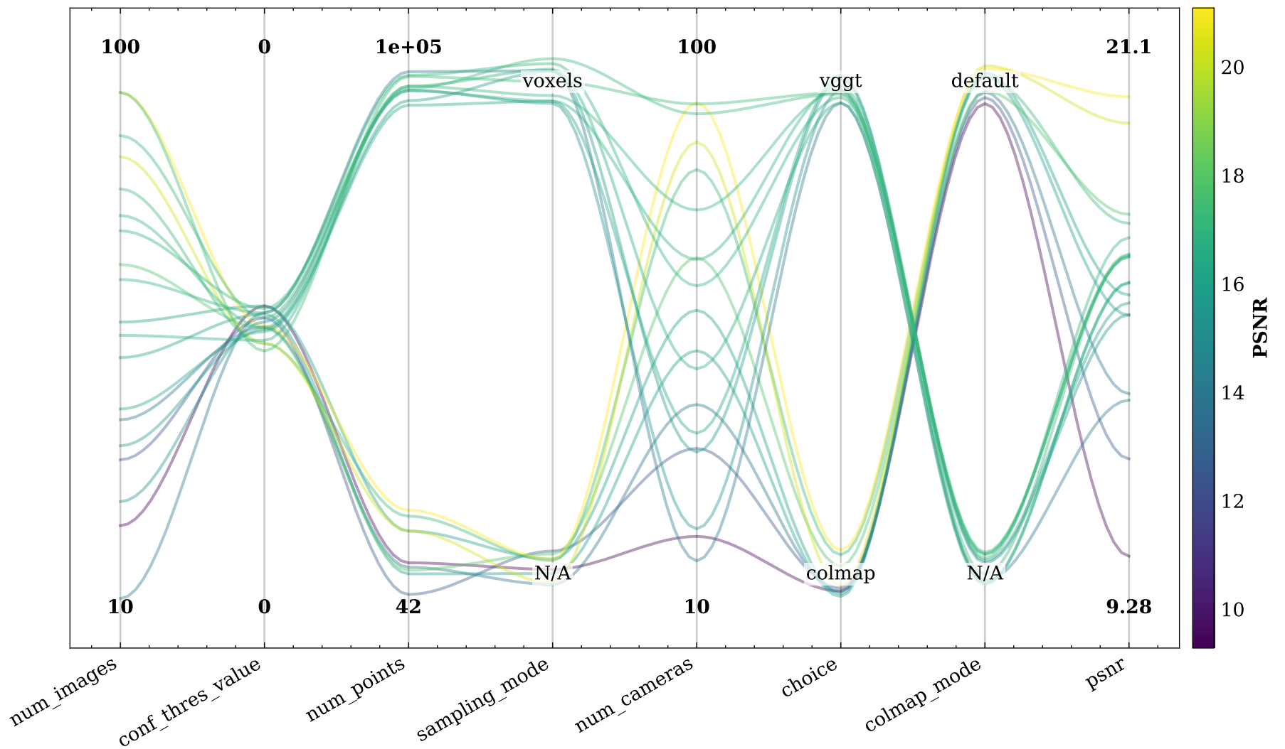
Parallel Coordinate Plot: Parameters vs PSNR
