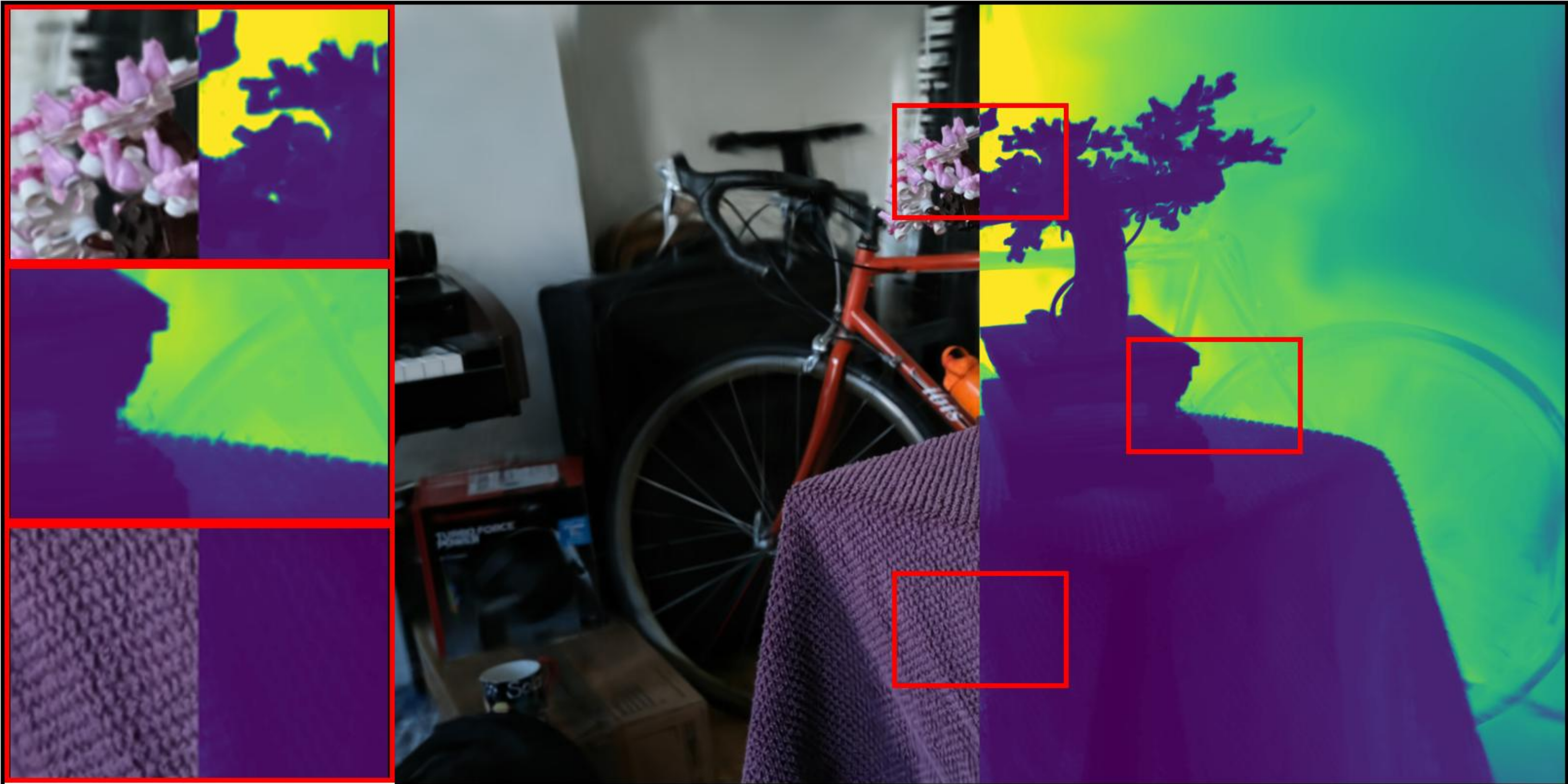
bonsai: VGGT | | depth_lambda=0.0 PSNR: 26.10 | LPIPS: 0.2117 | SSIM: 0.8380
