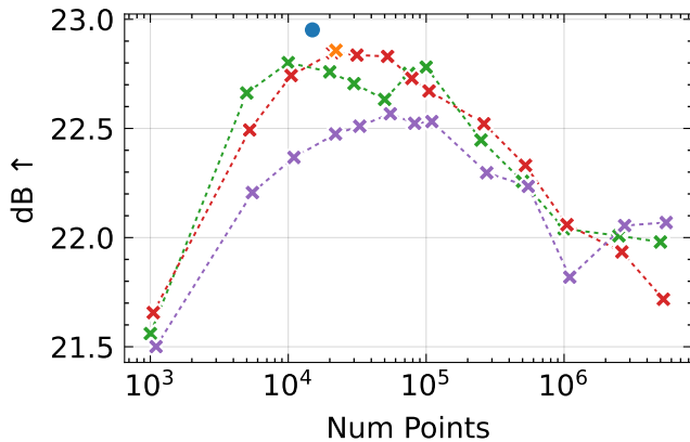
PSNR
