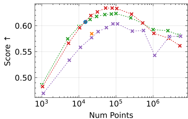
SSIM
