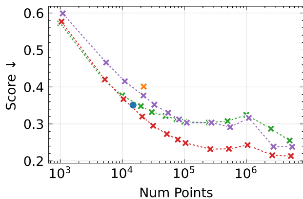
LPIPS
