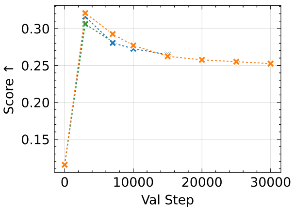
SSIM
