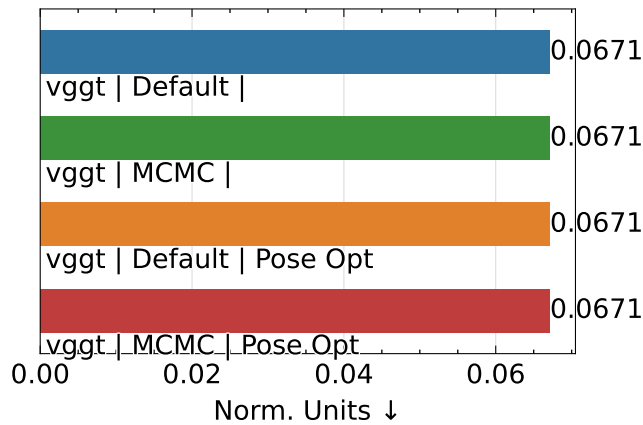
SSIM
