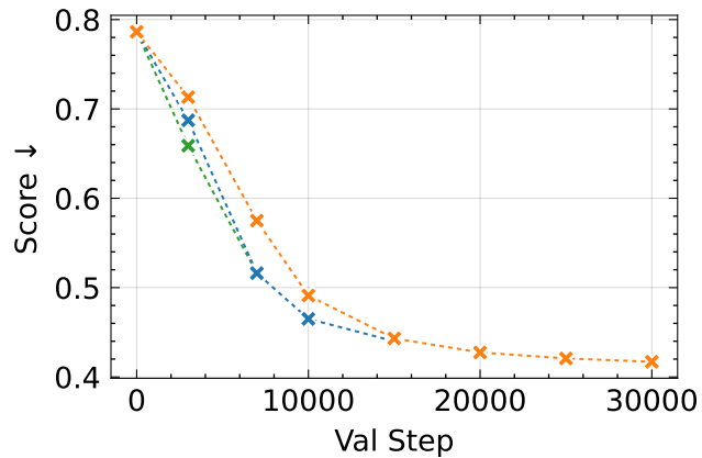
LPIPS
