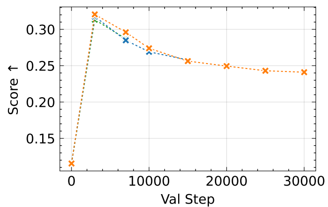
SSIM
