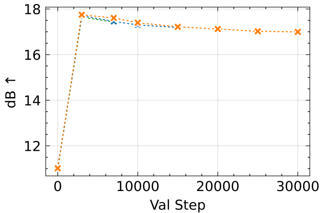
PSNR
