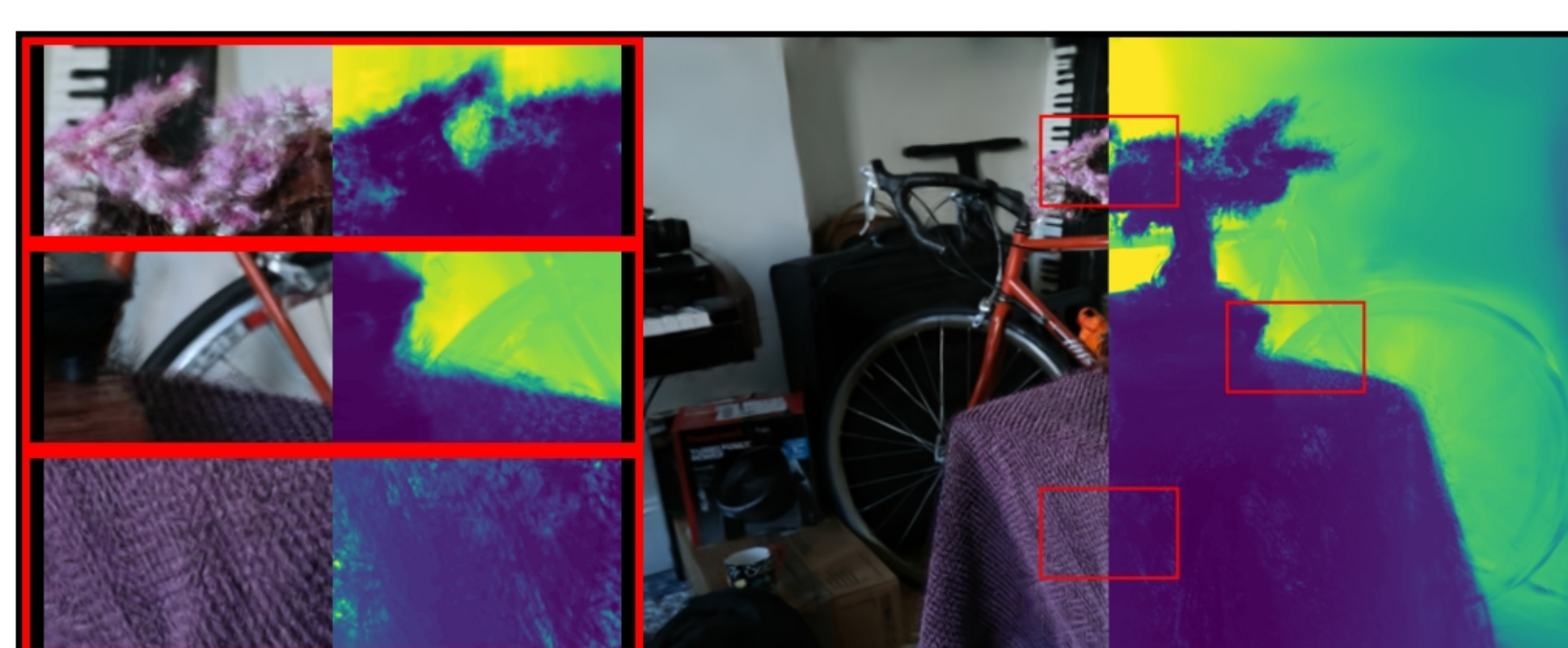
bonsai: VGGT | | PSNR: 17.73 | LPIPS: 0.4184 | SSIM: 0.5750
