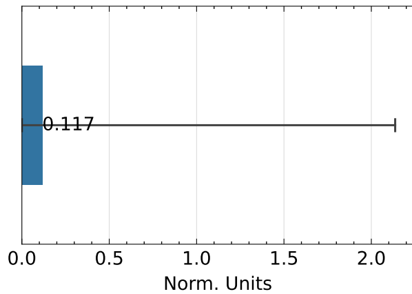
SSIM ↑
