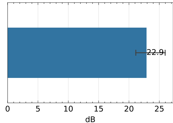
PSNR ↑
