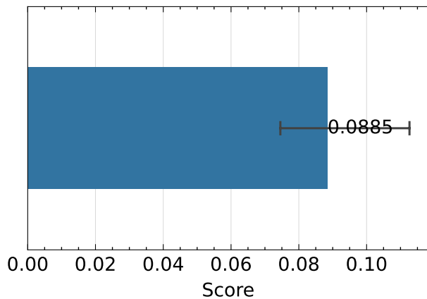
LPIPS ↓
