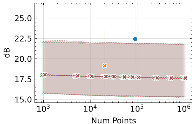
PSNR \uparrow
