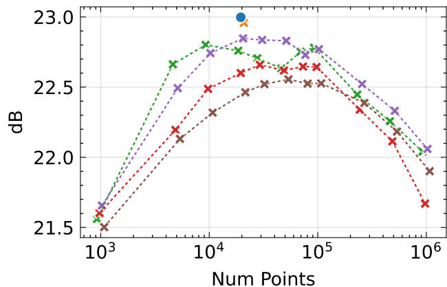
PSNR \uparrow
