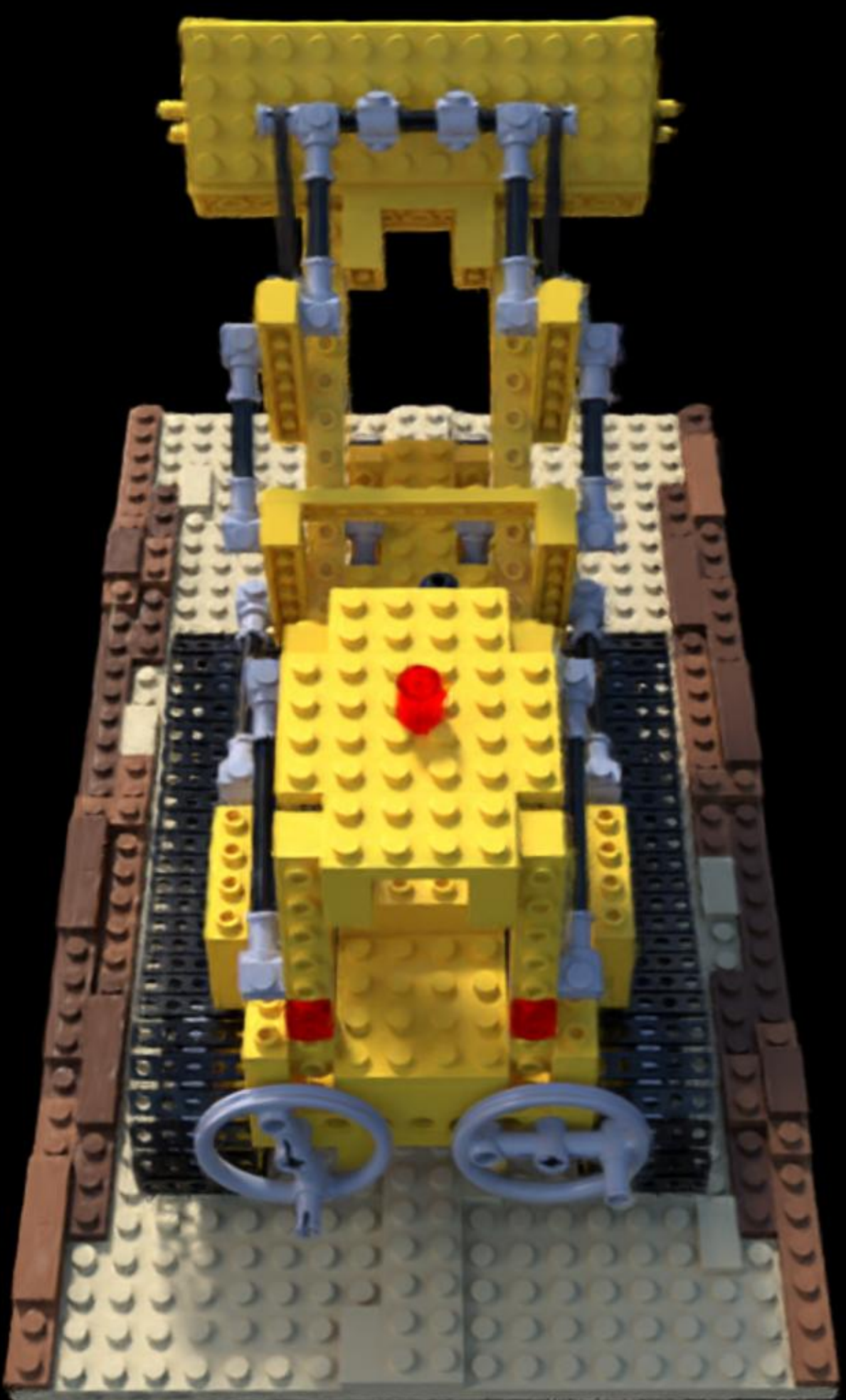
Config: VGGT | voxels | num_points=87000 PSNR: 20.20 | LPIPS: 0.1060 | SSIM: 0.7610
