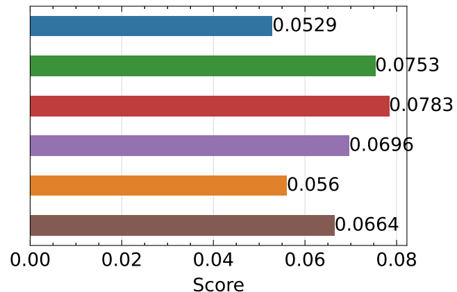
LPIPS ↓
