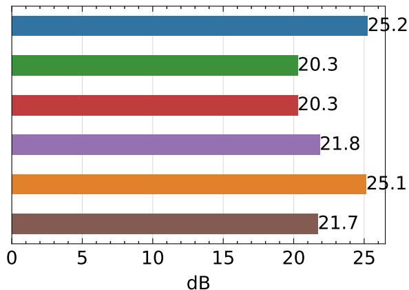
PSNR ↑
