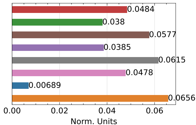
LPIPS ↓
