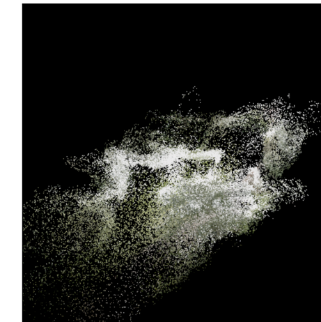
VGGT | | | (Zoom)
