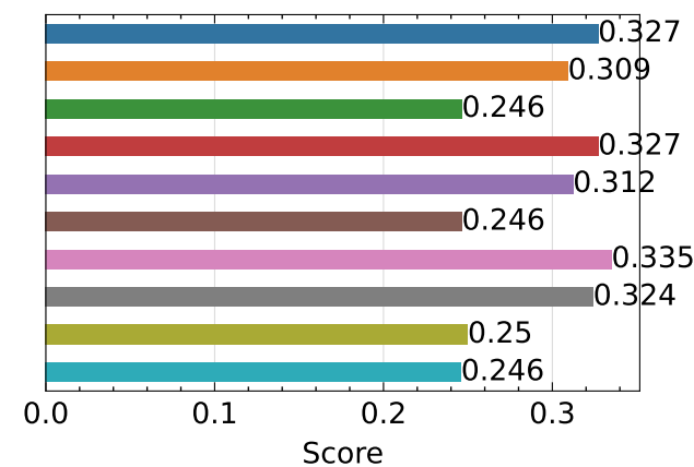
LPIPS ↓
