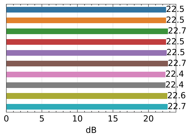
PSNR ↑
