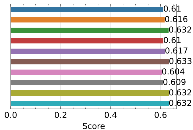
SSIM ↑
