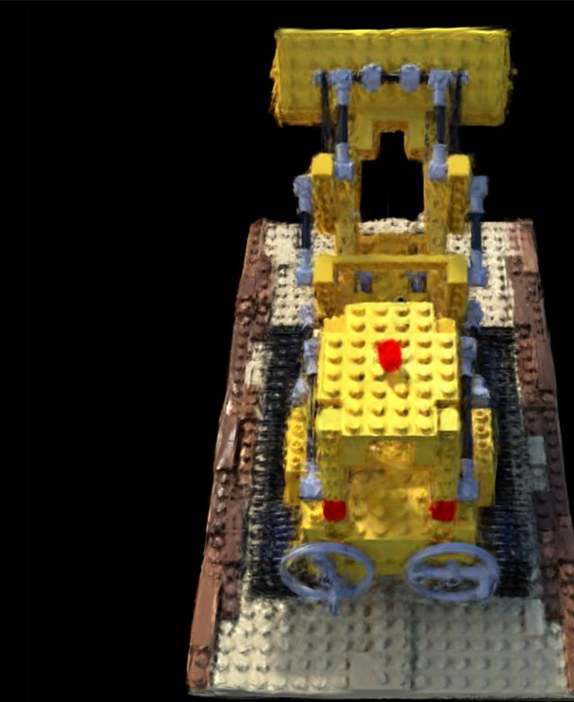
Config: VGGT | num_images=100 PSNR: 14.98 | LPIPS: 0.2760 | SSIM: 0.6537
