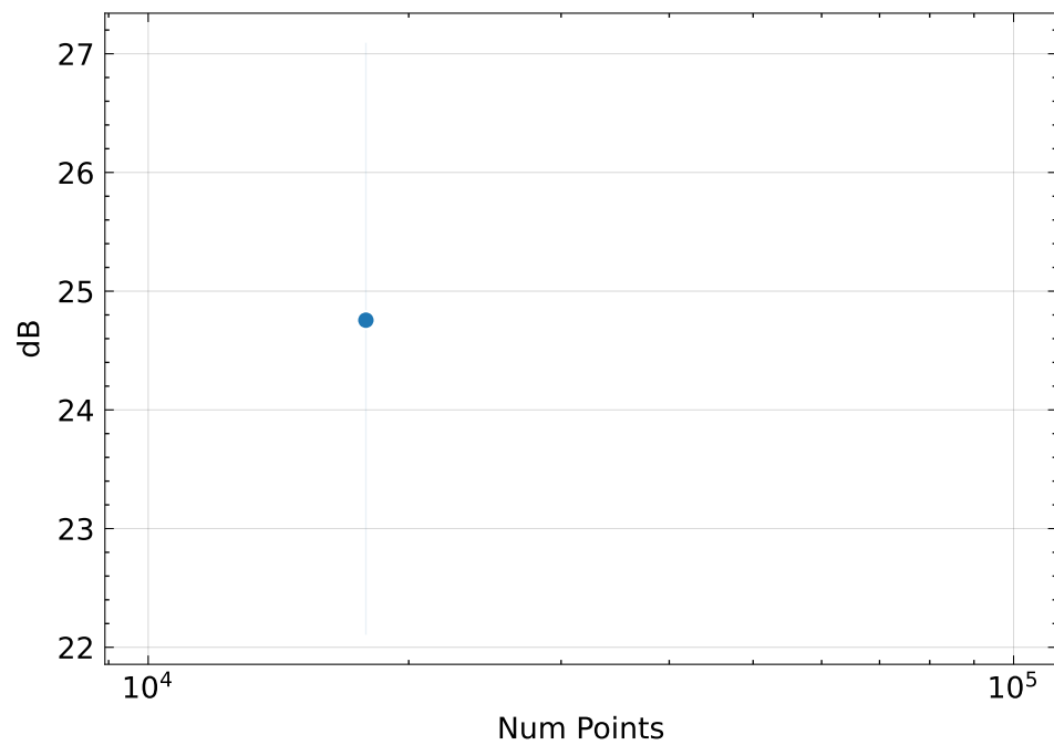
PSNR \uparrow
