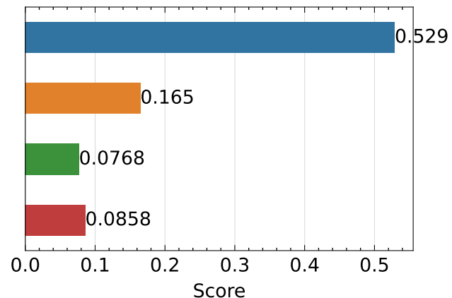
LPIPS ↓
