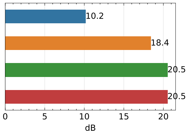
PSNR ↑
