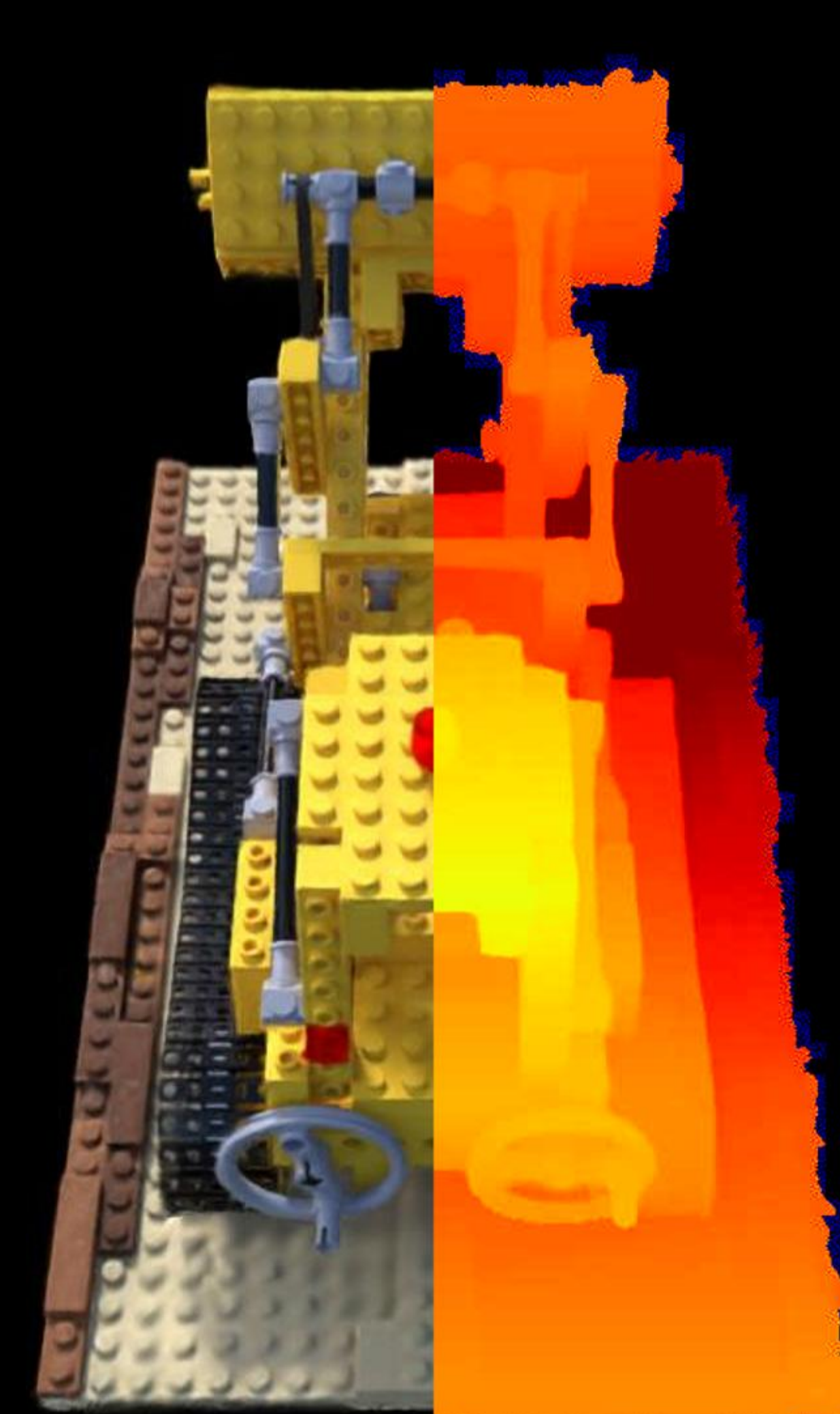
Config: VGGT | 1.0 | num_images=87 PSNR: 23.21 | LPIPS: 0.1075 | SSIM: 0.8370
