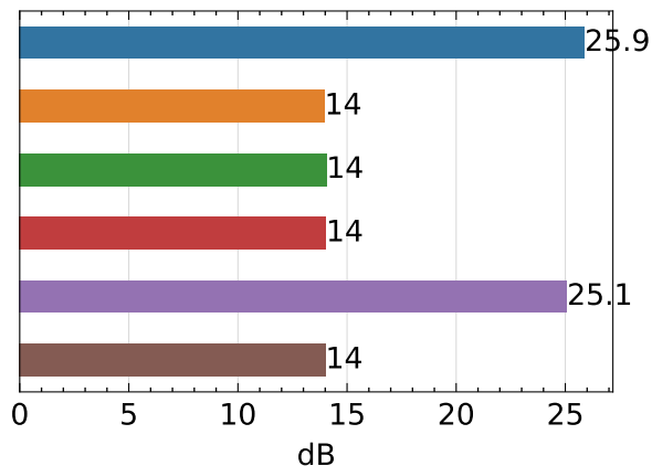
PSNR ↑
