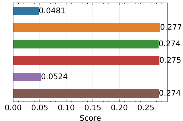
LPIPS ↓
