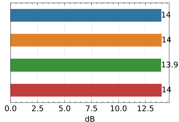
PSNR ↑
