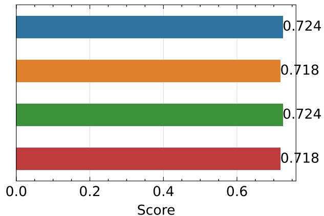
SSIM ↑
