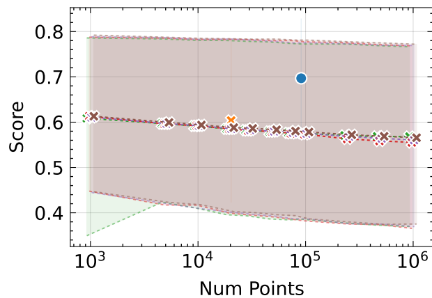
SSIM \uparrow - bonsai
