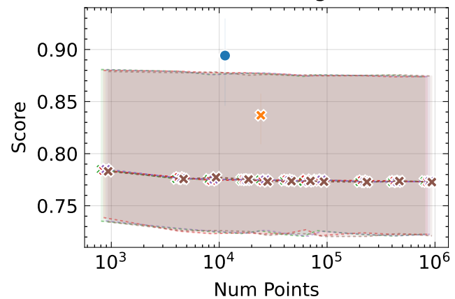
SSIM \uparrow - lego
