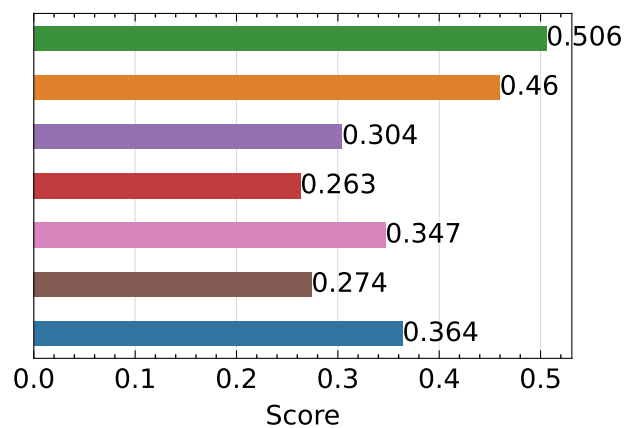
LPIPS ↓
