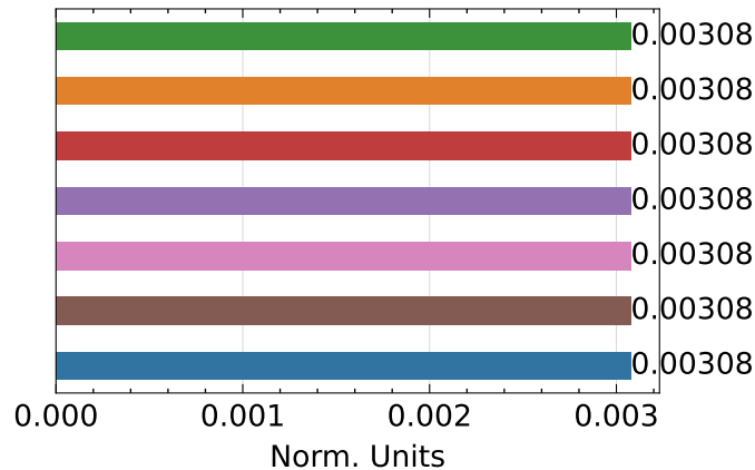
LPIPS ↓
