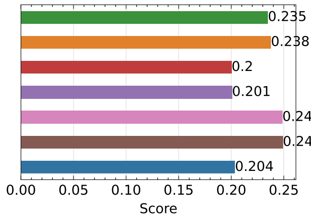
LPIPS ↓
