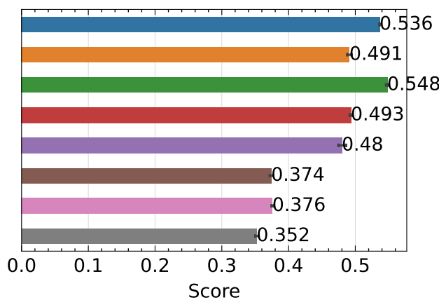
LPIPS ↓
