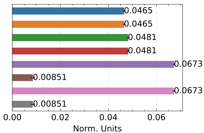
RTE ↓
