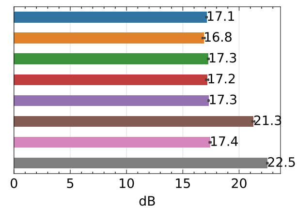
PSNR ↑
