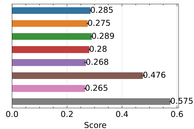
SSIM ↑
