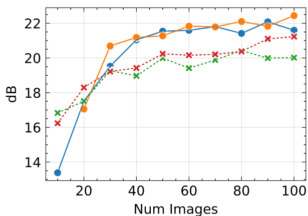
PSNR ↑
