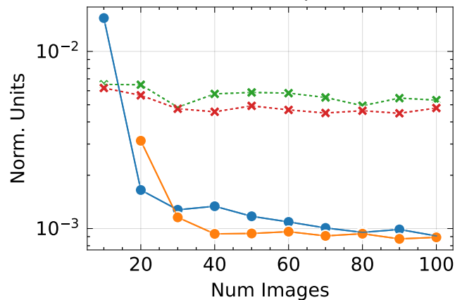
LPIPS ↓
