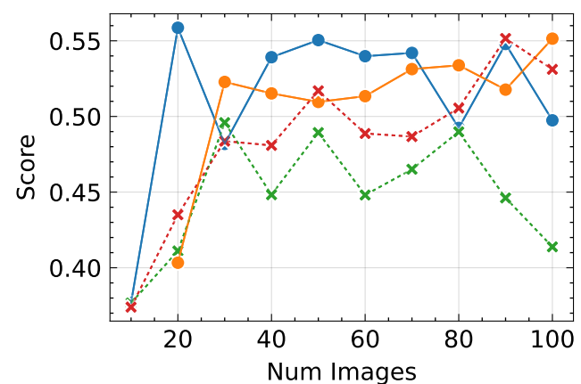
SSIM ↑
