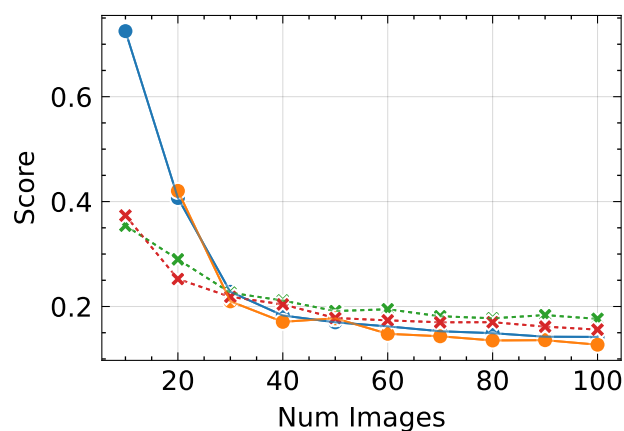
LPIPS ↓
