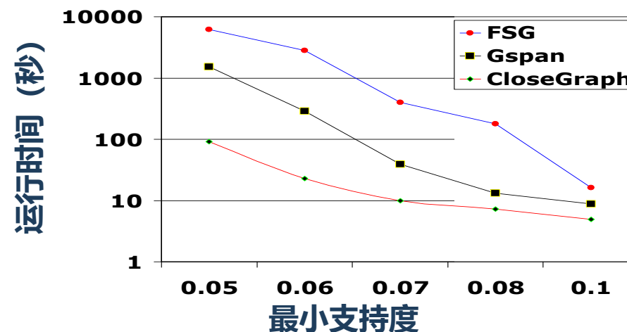
运行时间：频繁与闭
