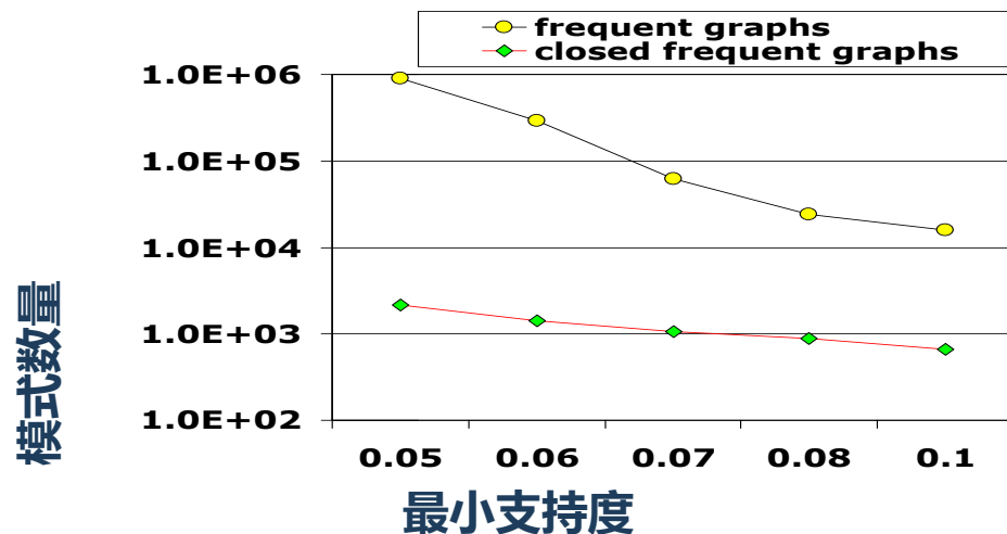
# 模式数：频繁与闭
