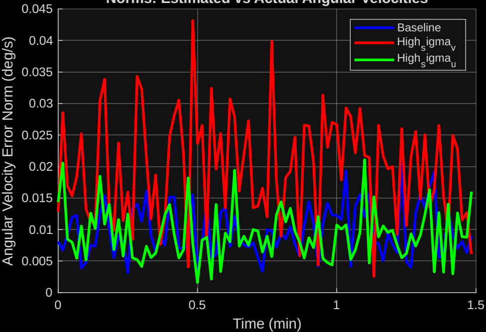
Norms: Estimated vs Actual Angular Velocities
