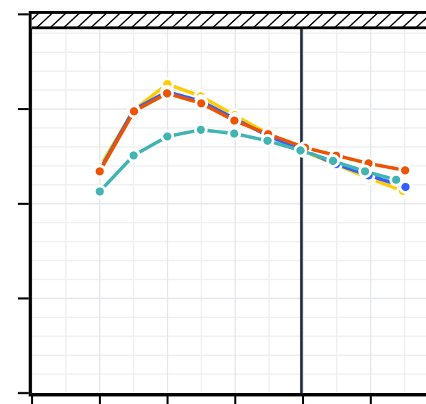
Torus
