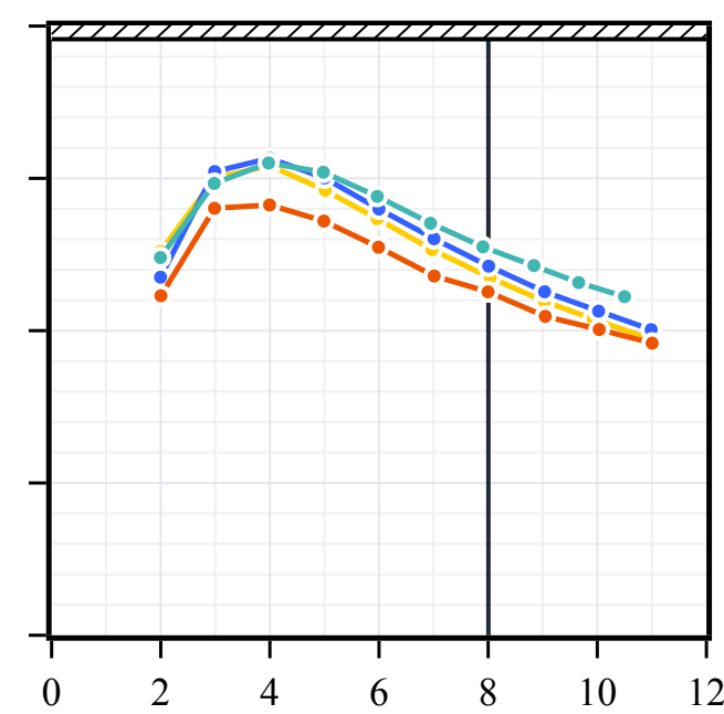
Torus
