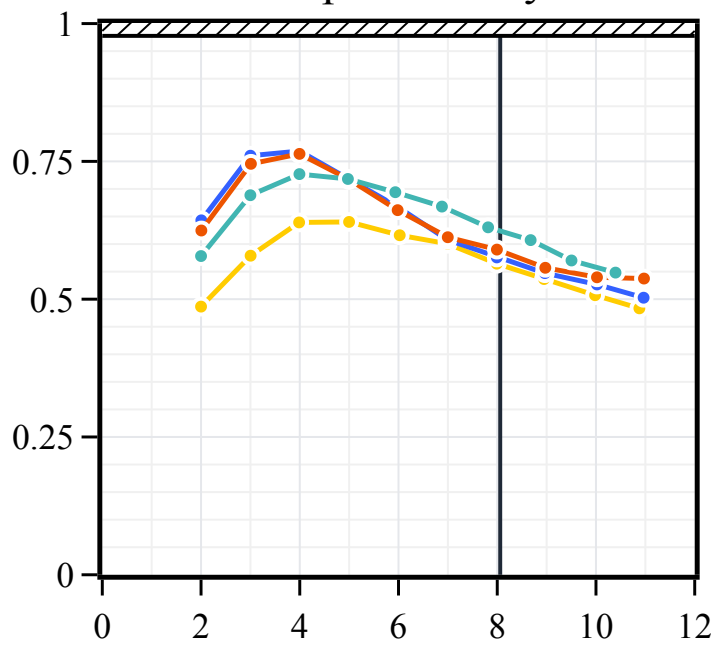
Deep Hierarchy
