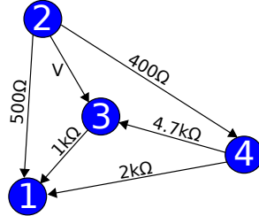
Abbildung 2.2: Beispiel: elektrischer Stromkreis als Graph.
