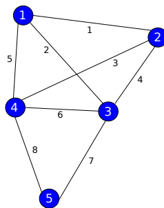
Abbildung 6.1: Beispiel eines Graphen.
