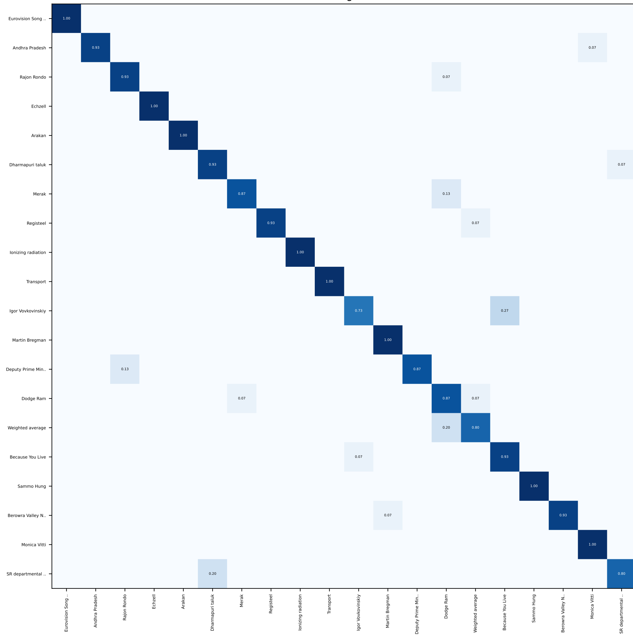
Padding OFF
