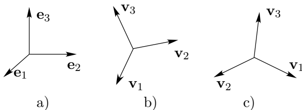
图 2 \mathbb{R}^3 中的取向
