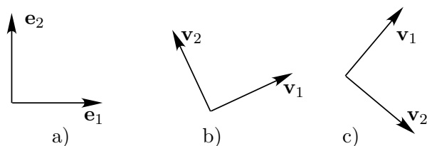
图 1 \mathbb{R}^2 中的取向
