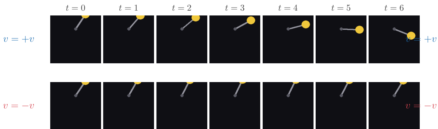
Pendulum
