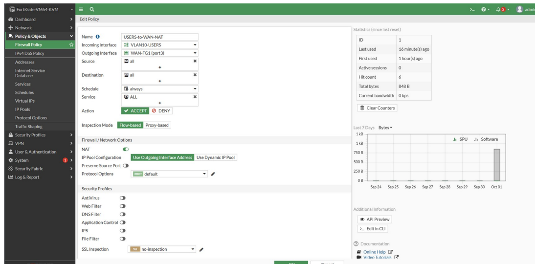
Figura 6. Política USERS-to-WAN-NAT con NAT habilitado en FortiGate 1.
