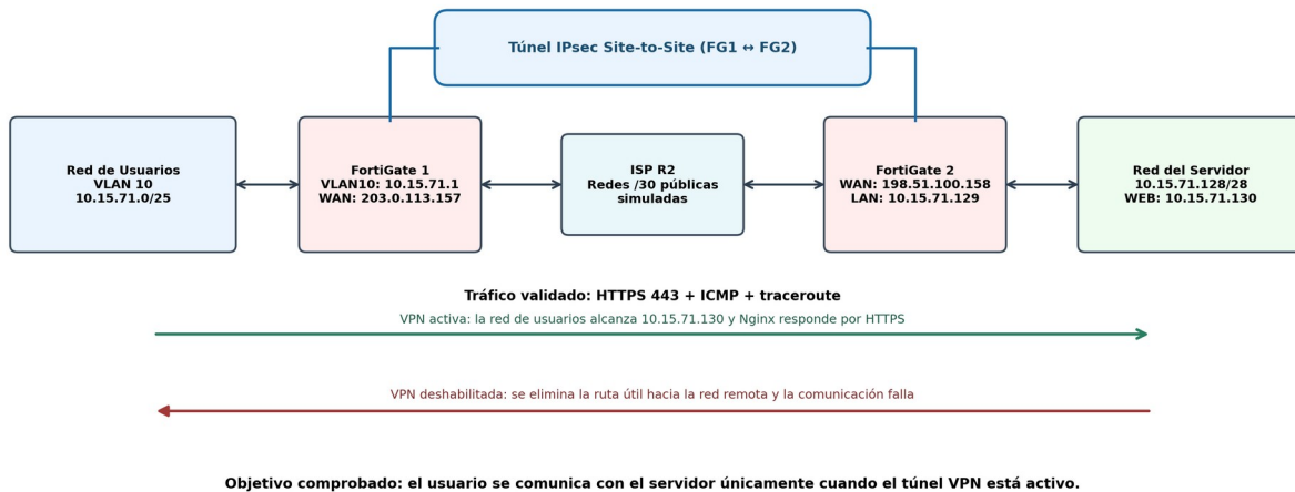
Figura 3. Flujo lógico del túnel VPN y comportamiento esperado con la VPN activa o deshabilitada.
