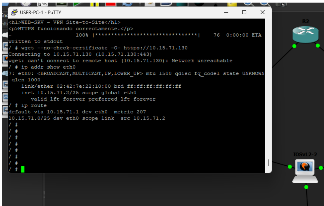
Figura 13. Dirección recibida por DHCP y ruta por defecto de USER-PC-1.
