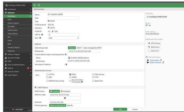
Figura 5. VLAN 10 y DHCP configurados sobre port2.
