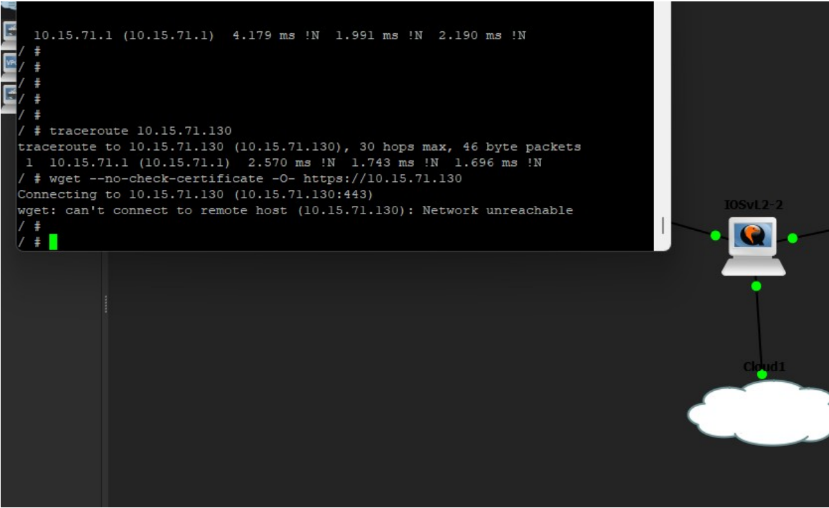
Figura 16. Traceroute y acceso HTTPS fallando con la VPN deshabilitada.
