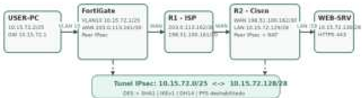
Figura 2. Diagrama logico del flujo entre la red de usuarios y el servidor por medio del tunel IPsec.
