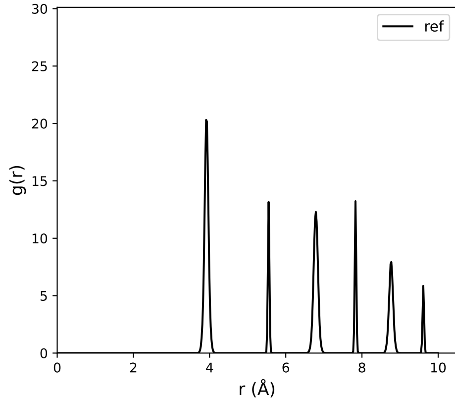
Si-Si
