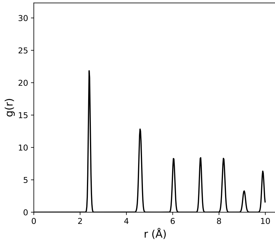
Si-Ge
