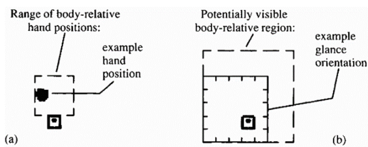
Figure 2.14. Environnement de test de Drescher [Dre91, Fig. 6.1]. Petit carré avec un point : corps du robot. Gros point : main qui peut bouger dans une région 3 \times 3 devant le corps. Région 5 \times 5 : champ visuel qui peut bouger dans la grille 7 \times 7 .
