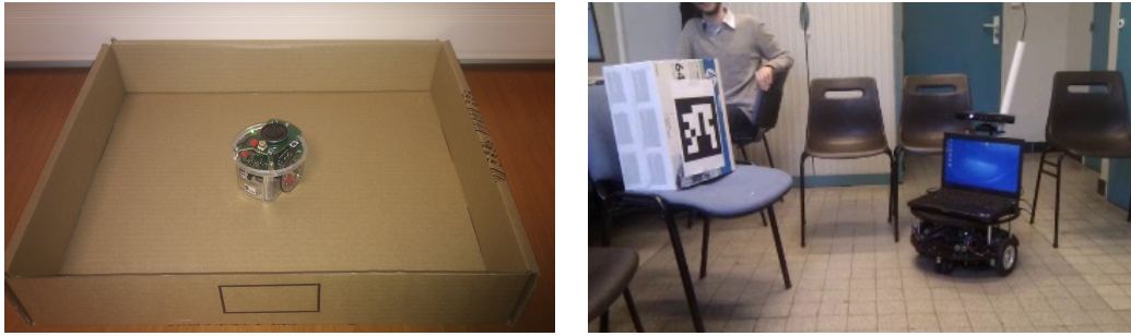
Figure 3.13. Gauche : robot e-puck répliquant l'expérimentation du Small Loop Challenge . Droite : robot Eddie répliquant l'expérimentation de la limule.
