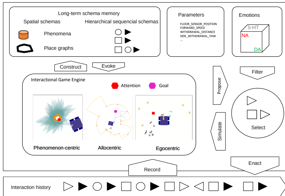
Figure 4.8. Représentation synthétique d'ECA pour Petitcat. Bas : historique des événements d'interaction, centre : moteur de jeu interactionnel , haut : mémoire à long terme des schémas, paramètres, système émotionnel.
