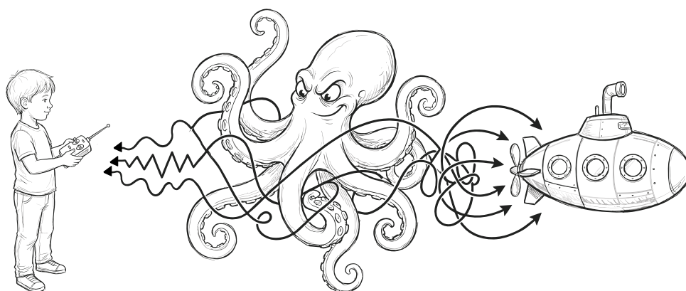
Figure 2.7. Métaphore du sous-marin de O'Regan et Noë [ON01]. Le cerveau serait dans la situation de la personne qui télécommande un sous-marin (qu'il ne voit pas), alors que toutes les connexions entrantes et sortantes ont été mélangées par un monstre marin.
