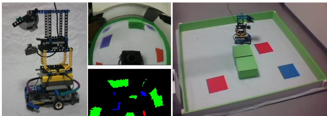
Figure 4.1. Gauche : robot disposant d'une caméra orientée vers un miroir sphérique offrant une vision panoramique. Centre : traitement d'image générant des événements de flux optiques. Droite : arène répliquant une expérimentation similaire à celle des requins décrite en Section 3.5.2.
