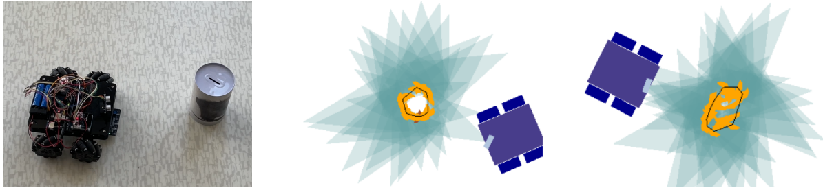
Figure 4.7. Apprentissage d'un phénomène représentant un objet cylindrique [GVKR22, Fig. 3]. Gauche : le robot observant l'objet. Centre : le phénomène caractérisé par les échos reçus depuis différentes positions autour de l'objet. Droite : phénomène obtenu avec deux objets cylindriques côte à côte.
