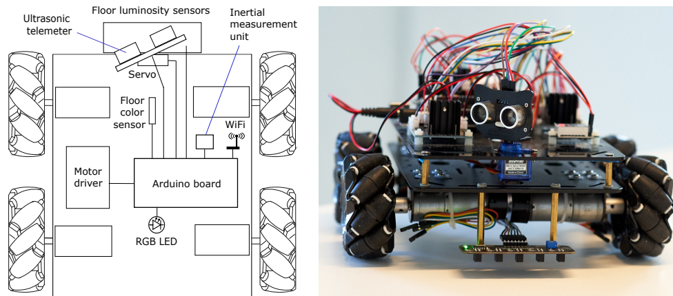
Figure 4.4. Robot Petitcat adapté de [GLR24, Fig. 7 et 8]. Connec- tée au PC de contrôle via wifi, la carte Arduino pilote l’énaction des décisions en commandant les effecteurs et capteurs : roues omnidirectionnelles, rotation de la tête, télémètre à ultrason, barre de capteurs de luminosité du sol, capteur de couleur du sol, carte inertielle, LED mul- ticolore.
