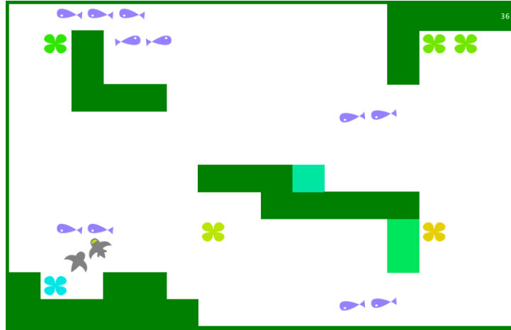
Figure 3.18. Environnement continu dynamique. Requins en bas à gauche : agents ECA. Poissons bleus : cibles mobiles. Cellules vert-foncées : murs. Cellules colorées : éléments de murs identifiable. Trèfles : algues traversables et identifiables visuellement.
