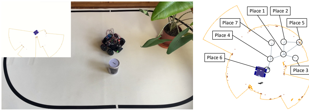
Figure 4.6. Expérimentation des cellules de lieu [GGR26, Fig. 1 et 3]. Gauche : conditions expérimentales. Encart : résultat d’une décision scan permettant de recueillir un profil télémétrique partiel du lieu 1 mettant en évidence la tirelire et le pot de fleur. Droite : graphe de places construits après 30 cycles d’interaction. Le robot est revenu proche du centre du lieu 6.
