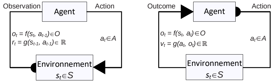
Figure 3.2. L'inversion du cycle d'interaction [GC14] montrant le début (puce noire) et fin (triangle noir) du cycle. Gauche : cycle des POMDP classiques. Droite : cycle inversé.
