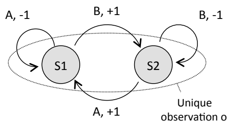
Figure 3.1. Un problème POMDP simple : le AB Problem adapté de [SJJ94]
