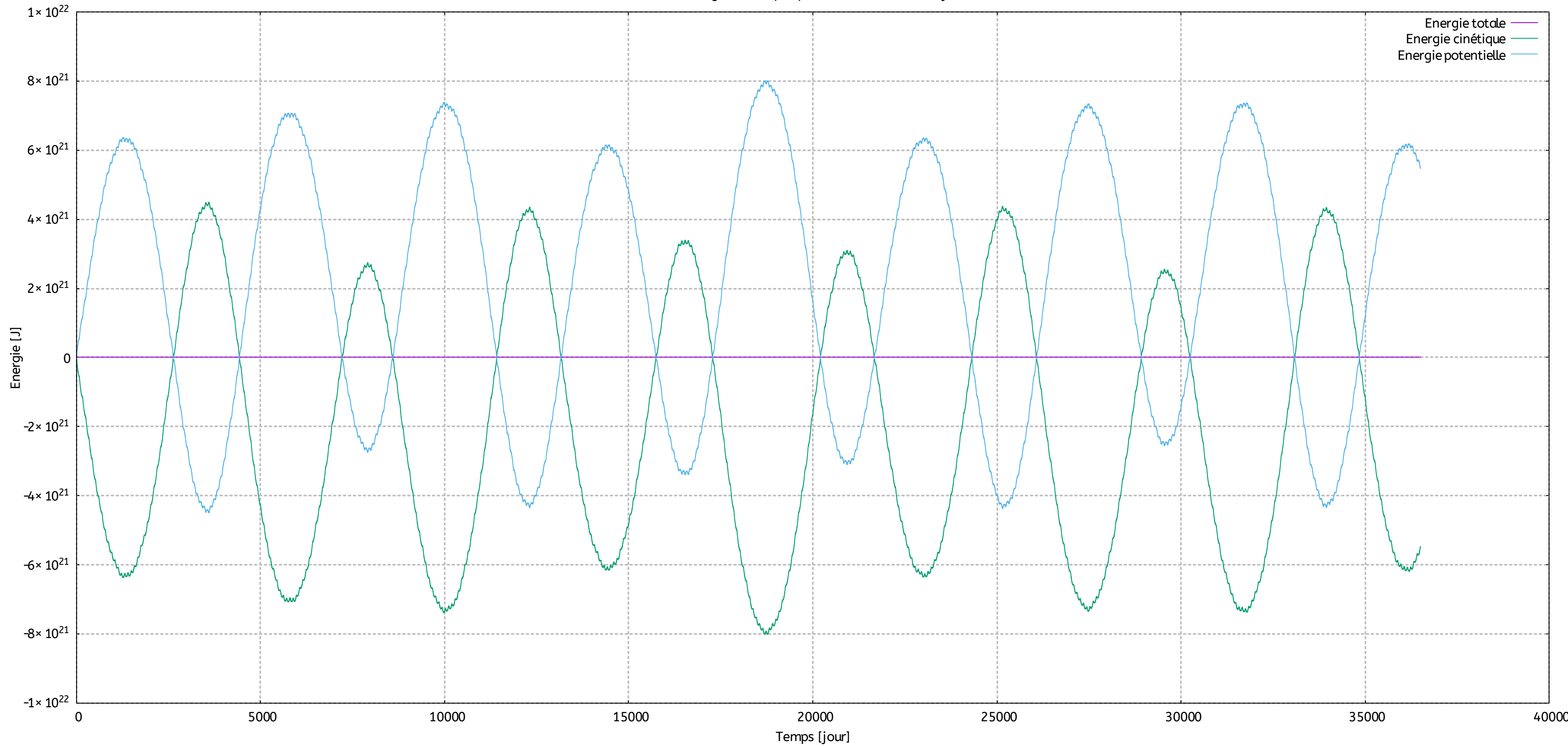
Evolution des énergies cinétique, potentielle et totale du système solaire
