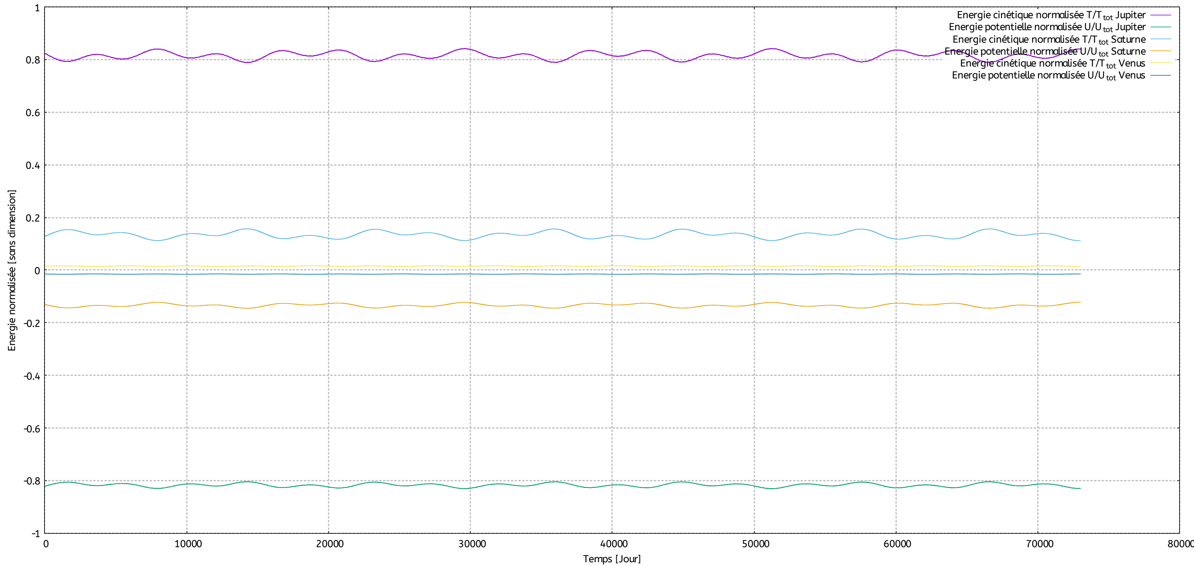
Evolution de l'énergie normalisée de Jupiter, Saturne et Vénus sur 200 ans
