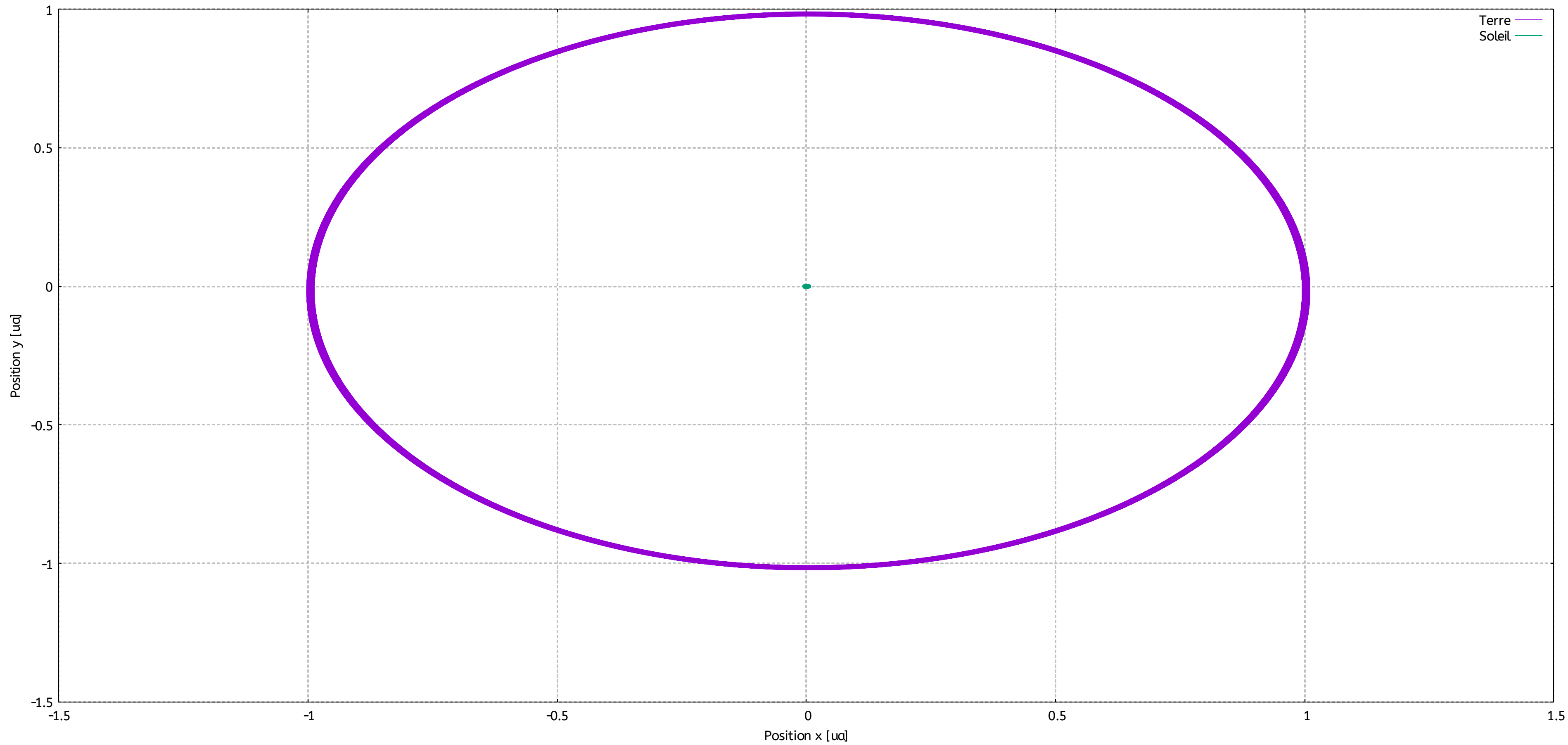
Trajectoire de la Terre autour du Soleil (système complet)
