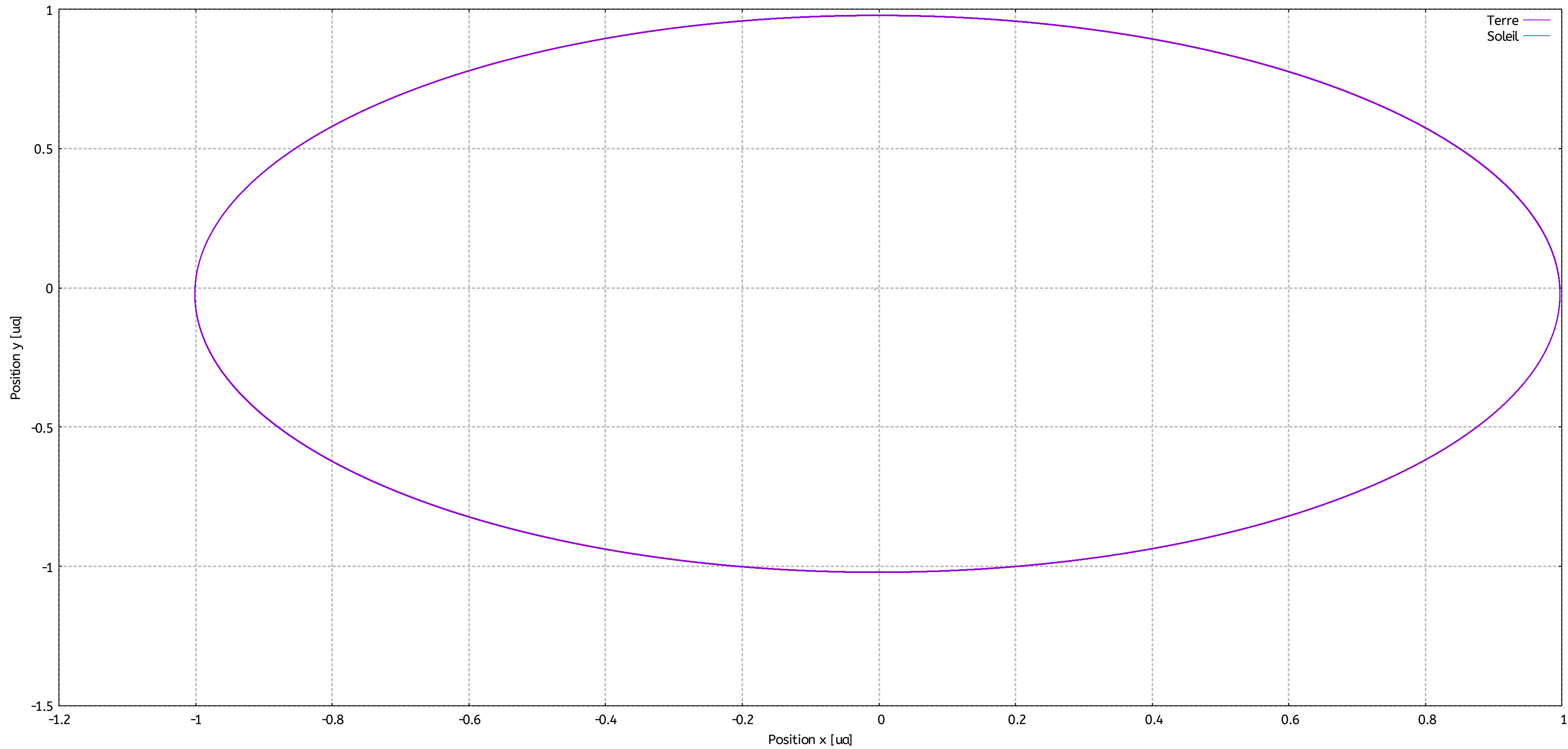
Trajectoire de la Terre autour du Soleil (système Terre/Soleil)
