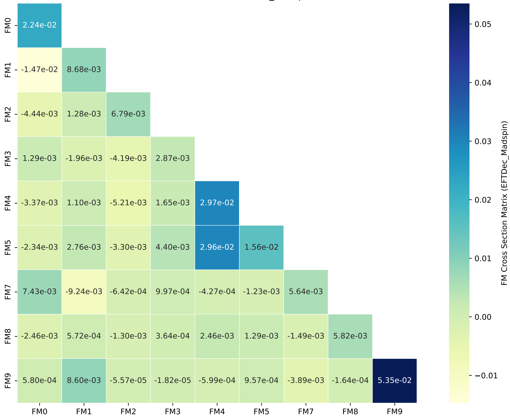
FM Cross Section Matrix (EFTDec_Madspin)
