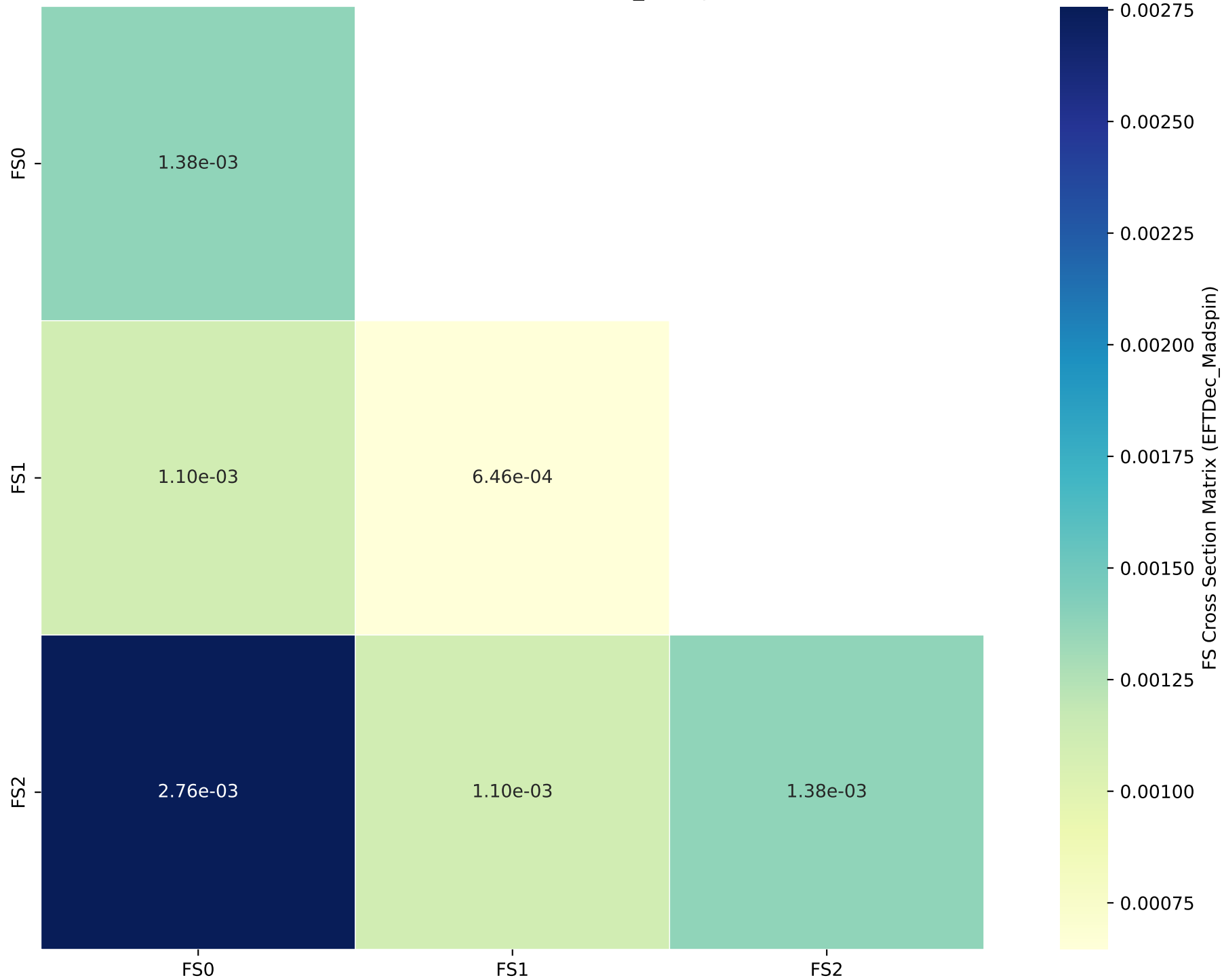
FS Cross Section Matrix (EFTDec_Madspin)
