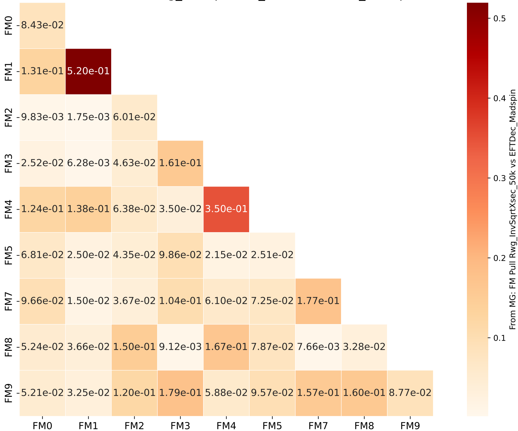
From MG: FM Pull Rwg_InvSqrtXsec_50k vs EFTDec_Madspin
