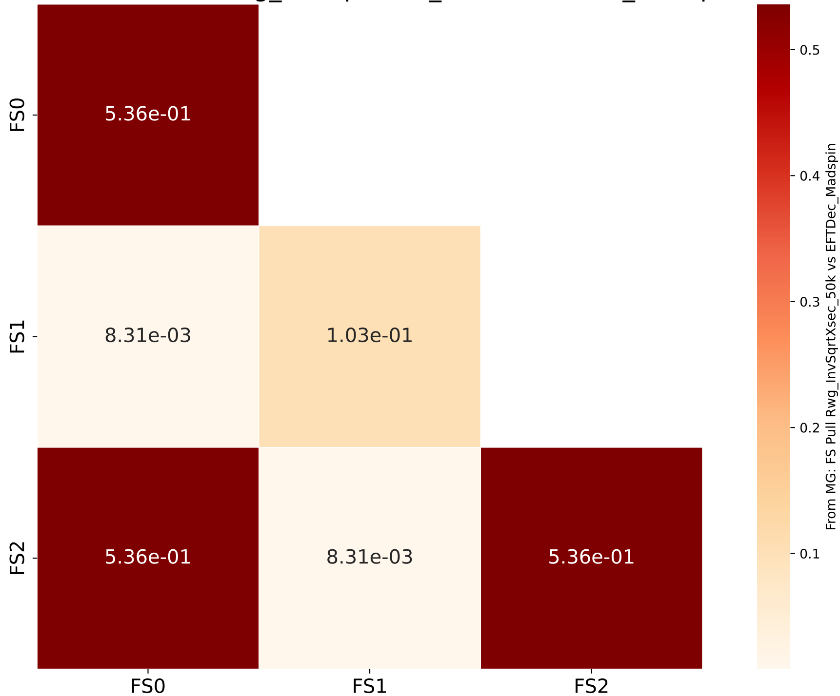
From MG: FS Pull Rwg_InvSqrtXsec_50k vs EFTDec_Madspin
